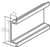
TH35-7.5 DIN Rail
