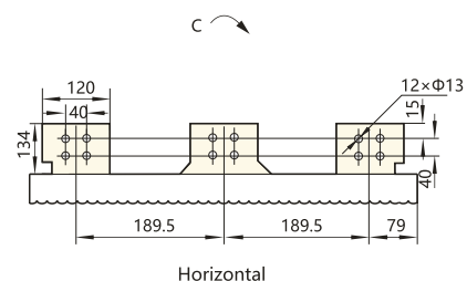
TIPO FIXO (3P)
