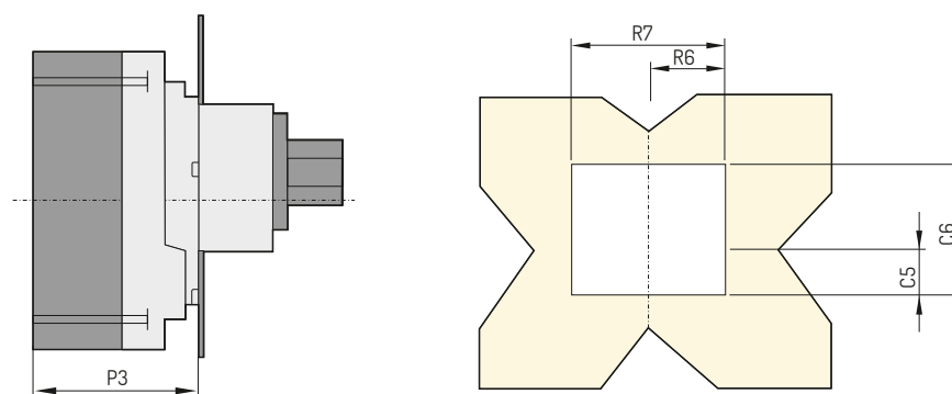
Orifício frontal (para disjuntores fixos ou extraíveis) [mm]
