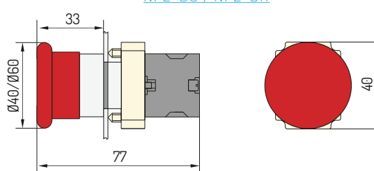
NP2-BC / NP2-BR
