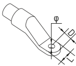
Terminal para cabo de cobre
