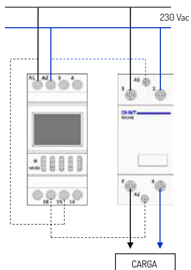
CABLAGEM ESTENDIDA (exemplo através de contactor modular)
