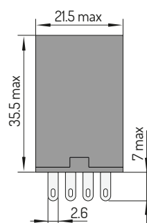
De encaixe, 4C
