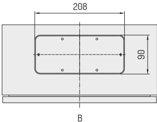
ENTRADA DE CABOS / Tipo B
