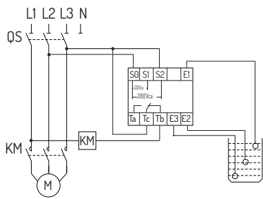
NJYW1-NL2 (Modo poço)
