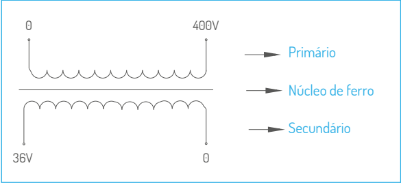
1 ENTRADA – 1 SAÍDA
