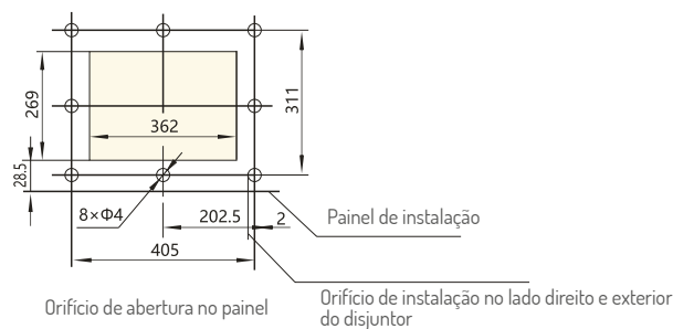
TIPO EXTRAÍVEL (3P)
