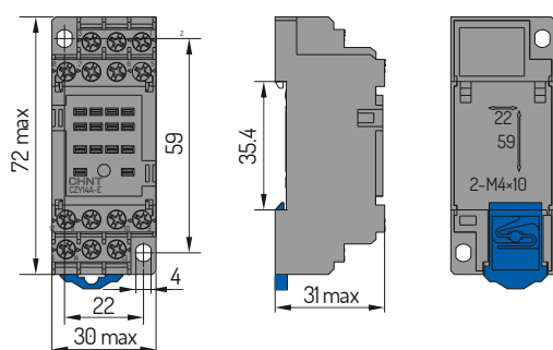
CZY14A-E
