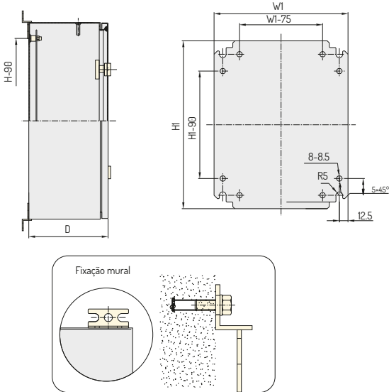
PLACA DE MONTAGEM ADJUNTA
