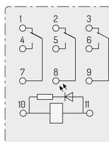
3C, com indicador
