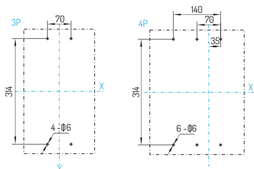
DIMENSÕES DE INSTALAÇÃO DA PLACA DE MONTAGEM (mm)
