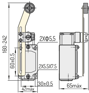
Serie YBLX-P1/120
