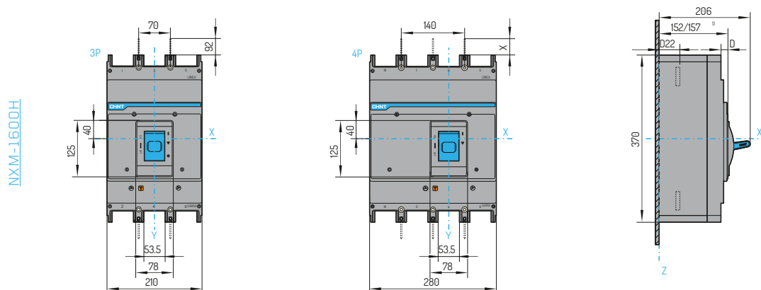
LIGAÇÃO FRONTAL, DIMENSÕES (mm)
