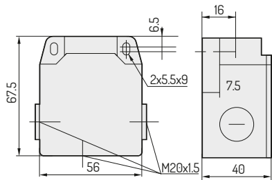
Serie YBLX-P1/100
