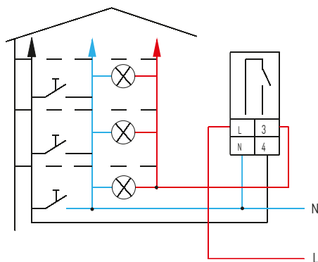
Conexão NJS3 (3 fíos)
