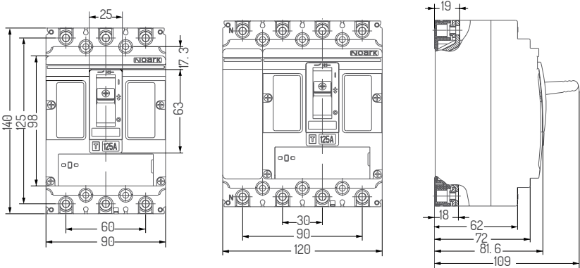
M1 (125)
