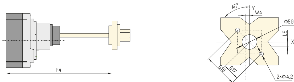
Orifício frontal (para disjuntores fixos ou extraíveis) [mm]
