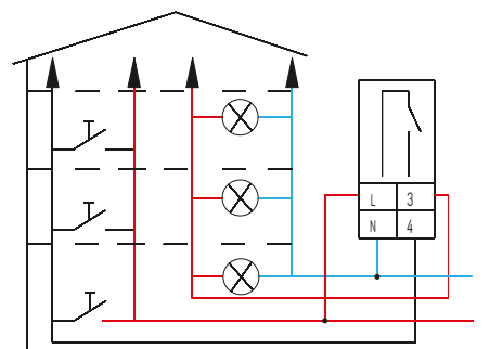
Conexão NJS3 (4 fíos)
