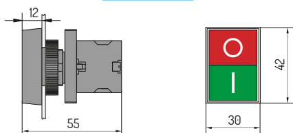
NP2-EL8325
