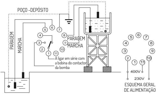
CNT2: Controlo de poço e depósito
