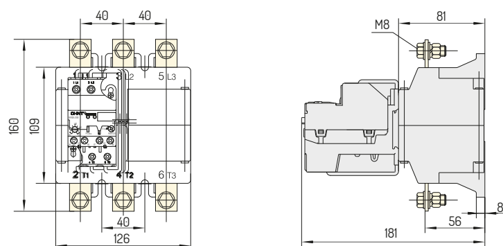
NRE8-200
