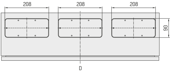
ENTRADA DE CABOS / Tipo D
