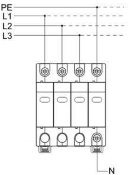
Ex9UE1+2 12.5 3PN 275
