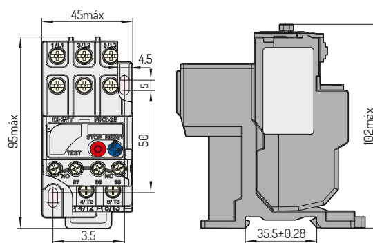
NR2-25 com MB-2
