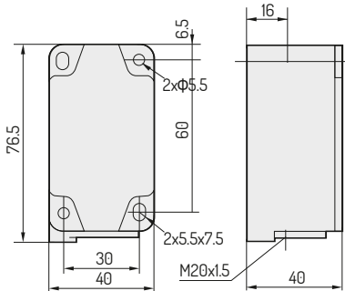
Serie YBLX-P1/120
