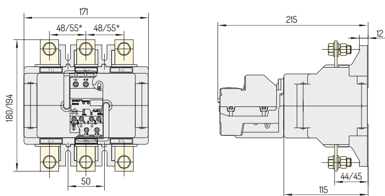
NRE8-630
