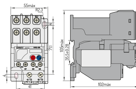
NR2-36 com MB-3
