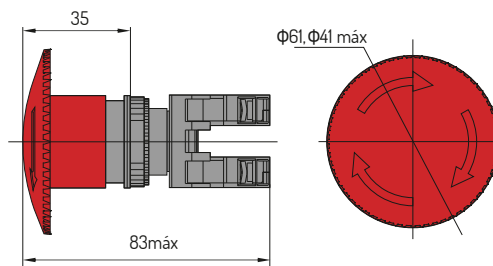
NP8-Z5
