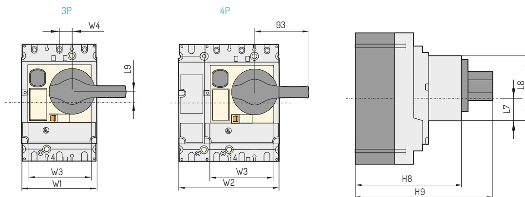
Orifício frontal (para disjuntores fixos ou extraíveis) [mm]
