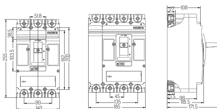
M3 (400)
