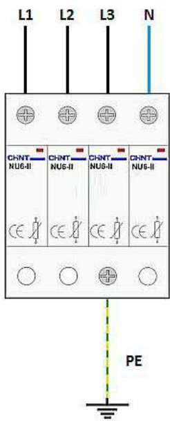
NU6-II-4
