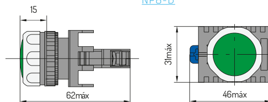
NP8-D
