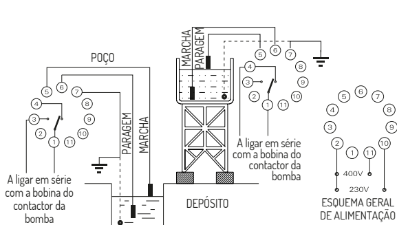
CNT1: Controlo de poço e depósito
