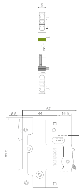
DIMENSÕES GERAIS E DE MONTAGEM (mm)
