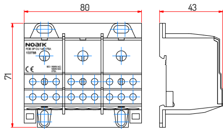
PDB 3P CU 1x6 175A
