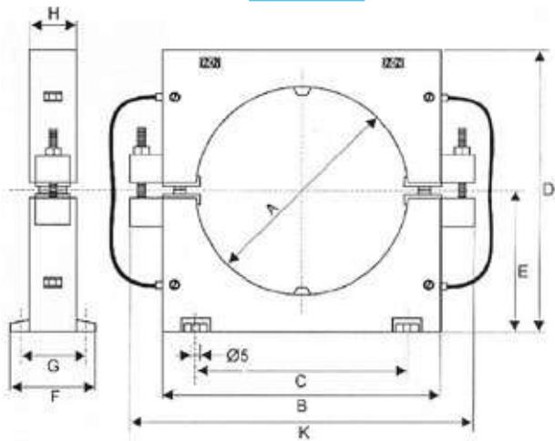
TTC-110A
