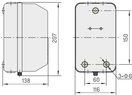
DIMENSÕES GERAIS E DE MONTAGEM
