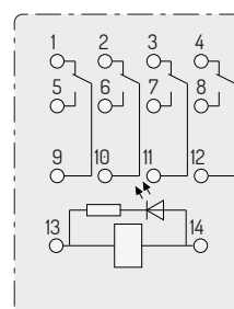
4C, com indicador
