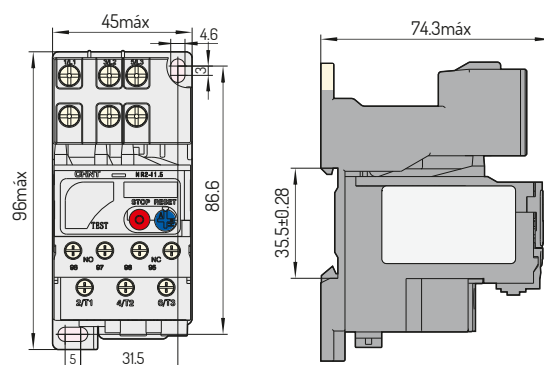
NR2-11.5 com MB-1
