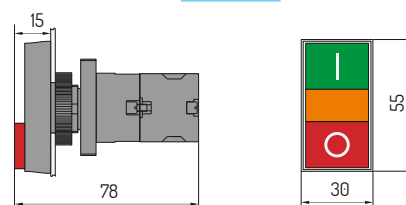
NP2-8_6_
