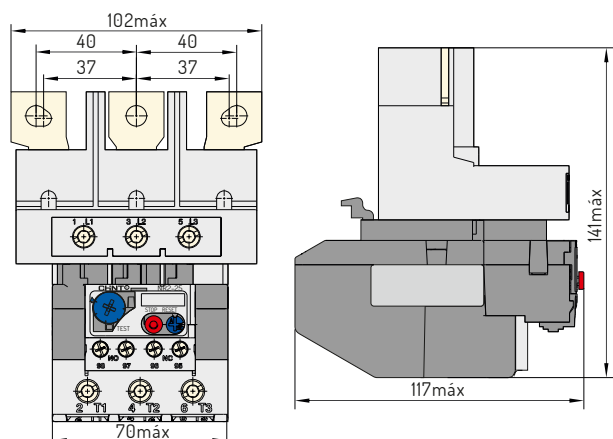
NR2-150 (combinado com NC2)
