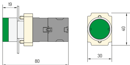
NP2-BW3_6_
