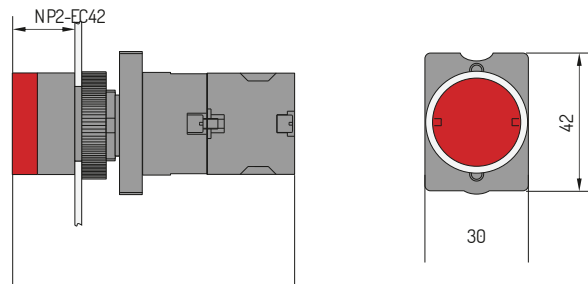
NP2-EW
