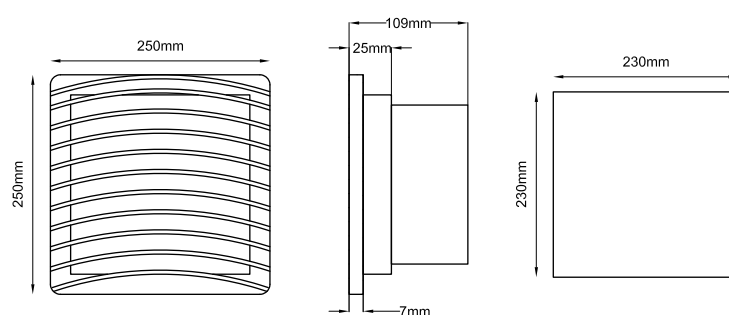
NTF1-160.230/NTF1-160.300
