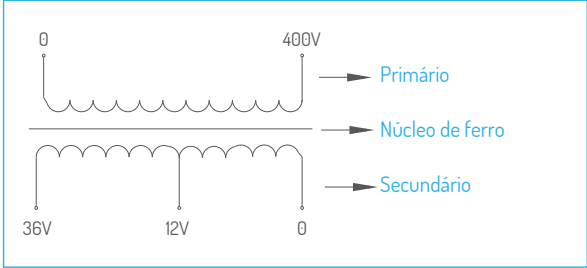
1 ENTRADA – 2 SAÍDAS
