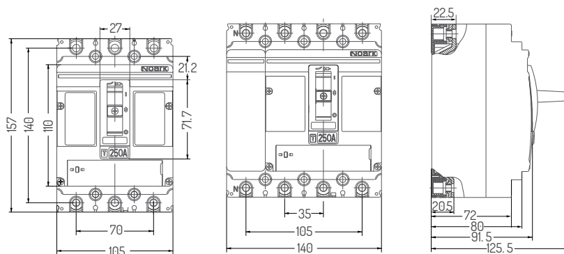
M2 (250)
