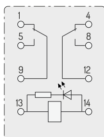
2C, com indicador
