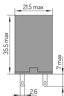
De encaixe, 2C
