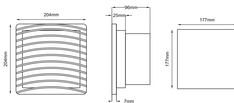
NTF1-160.230/NTF1-160.300
