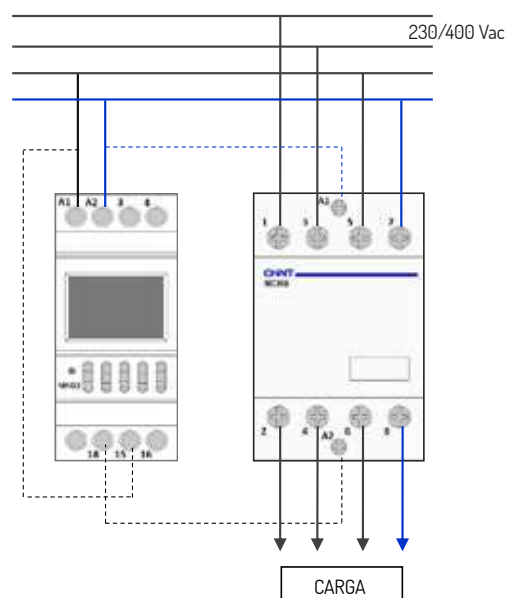
CABLAGEM TRIFÁSICA (exemplo através de contactor modular)
