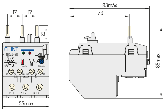
NRE8-40/F
