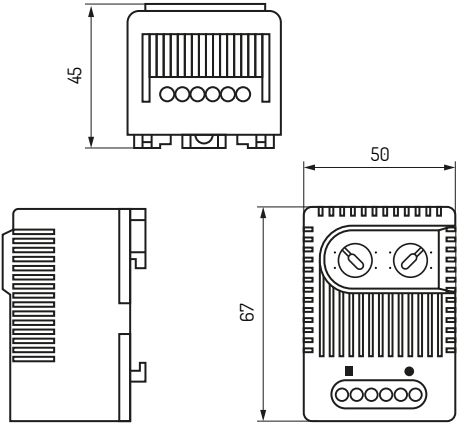
Modelo NTK3-**
